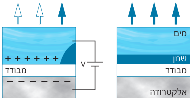
איור 11: מבט צד על שני מצבי פיקסל מונו-כרומטי המבוסס על הרטבה חשמלית. מימין האור המוחזר הוא כחול (כצבע שכבת השמן) ללא מתח חשמלי, ומשמאל האור הוא לבן (כצבע שכבת המבודד) עם הפעלת מתח.
