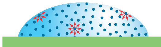
איור 2: המולקולות בתוך הטיפה נמשכות באופן שווה לכל הכיוונים, ואילו המולקולות על שפת הטיפה נמשכות פנימה אל שכנותיהן - וזה המקור למתח פנים.
