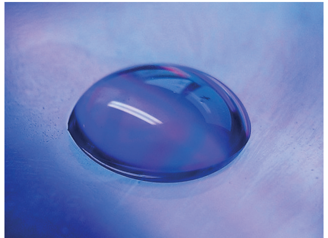
איור 1 א': טיפת מים על משטח בעל קיטוביות (פולריות) גבוהה, כגון זכוכית או מתכת. הטיפה משתטחת וההרטבה רבה. צילמה: Betty Winter
