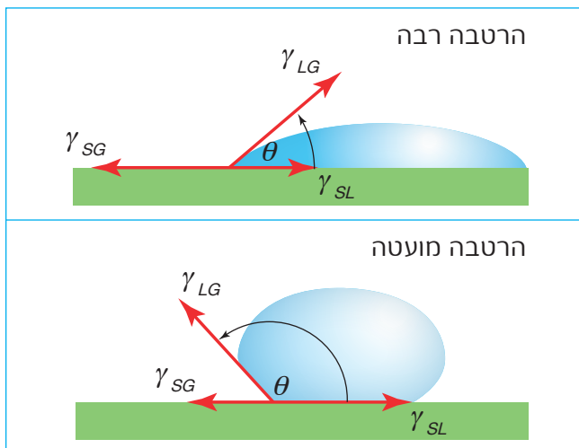
איור 3: דרגות שונות של הרטבה. למעלה ההרטבה היא רבה וזווית המגע קטנה. למטה ההרטבה מועטה וזווית המגע גדולה. אם רושמים משוואת כוחות על פי השרטוט מקבלים את משוואת יאנג.
