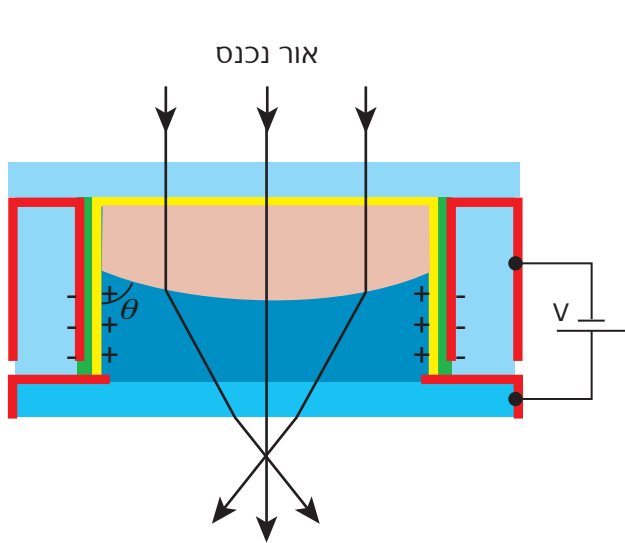
איור 9: ימין: תאור סכמאטי של חתך עדשה אופטית המורכבת מטיפת מים בתווך של שמן. כאן לא מופעל מתח חשמלי והטיפה הכדורית מפזרת אור בגלל מקדם השבירה הגבוה יותר של השמן ביחס למים (לפי חוק סנל). שמאל: כאן מופעל מתח חשמלי, בהשפעתו מתקערת טיפת המים בשמן וממקדת אור שעובר דרכה.
