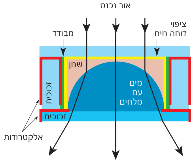
איור 9: ימין: תאור סכמאטי של חתך עדשה אופטית המורכבת מטיפת מים בתווך של שמן. כאן לא מופעל מתח חשמלי והטיפה הכדורית מפזרת אור בגלל מקדם השבירה הגבוה יותר של השמן ביחס למים (לפי חוק סנל). שמאל: כאן מופעל מתח חשמלי, בהשפעתו מתקערת טיפת המים בשמן וממקדת אור שעובר דרכה.
