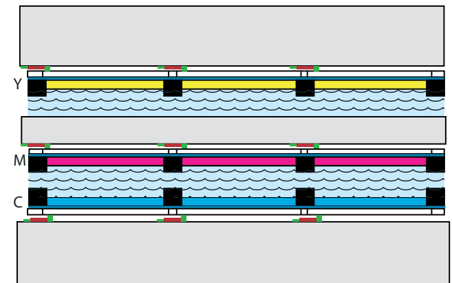
איור 13: פיקסל הרטבה חשמלית צבעוני שבו שכבות שמן בצבעים שונים ממוקמות זו על גבי זו, צהוב Y , מג'נטה M , ציאן C .
