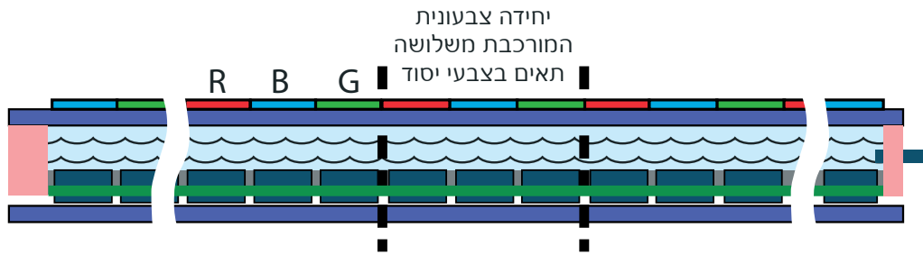
איור 12: פיקסל הרטבה חשמלית צבעוני שמורכב מחיבור של שלושה פיקסלים מונו-כרומטיים בצבעי היסוד האופטיים אדום R , כחול B , ירוק G .
